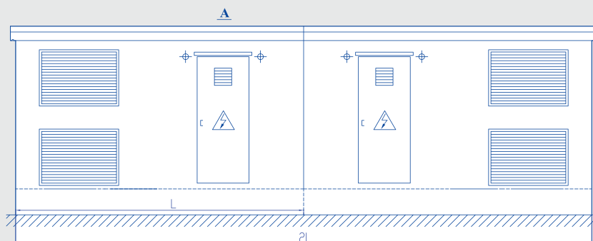
2КТПБ – параллельная стыковка блоков
