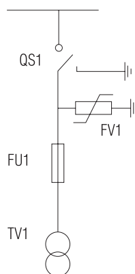
Трансформатор напряжения
