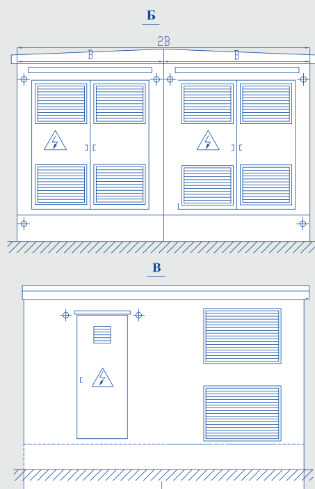
2КТПБ – параллельная стыковка блоков
