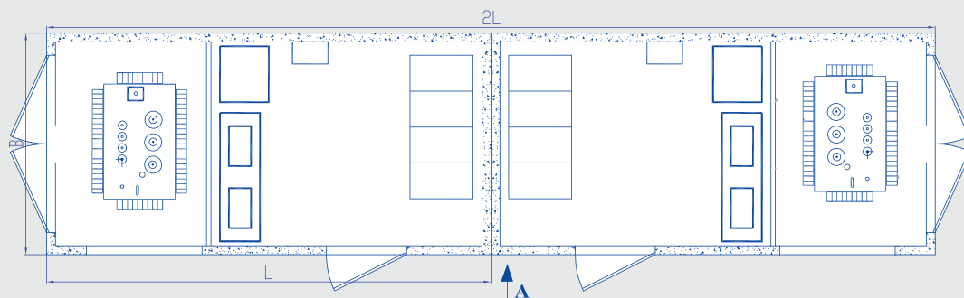
2КТПБ – последовательная стыковка блоков**
