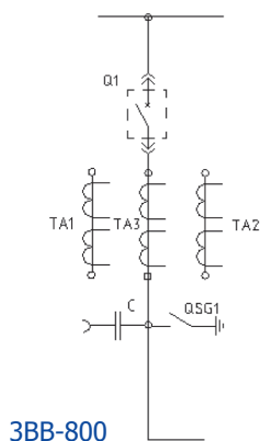
Секционный выключатель
