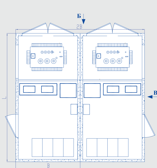
2КТПБ – параллельная стыковка блоков
