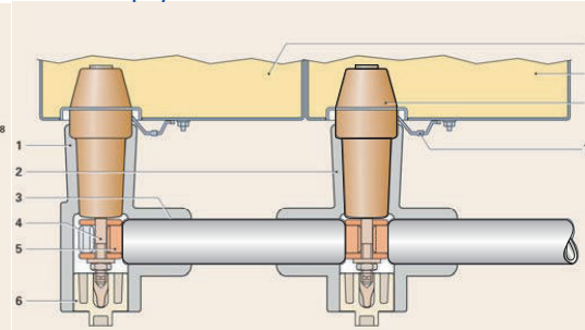
Соединение сборных шин соседних панелей (общий вид при снятии крышки)
